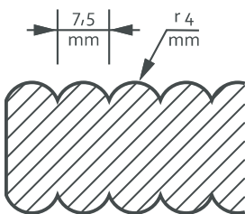
1:1 Querschnitt
